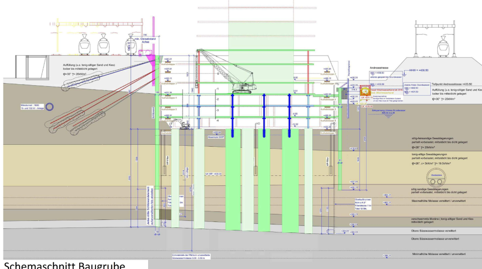
Schemaschnitt Baugrube
