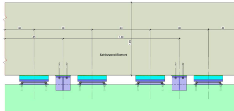
Grundriss Deckenrand Spriessdecke mit Flachpressen und Entkoppelungslager
