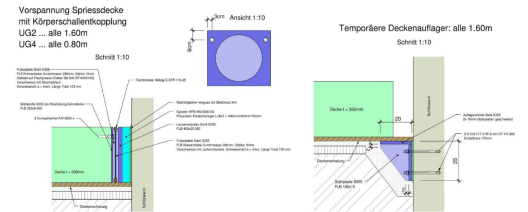
Schnitt Deckenrand Spriessdecke
