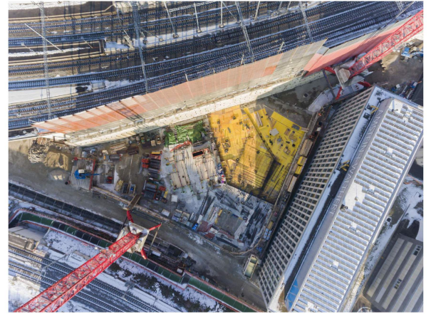
Vogelperspektive Baustelle
