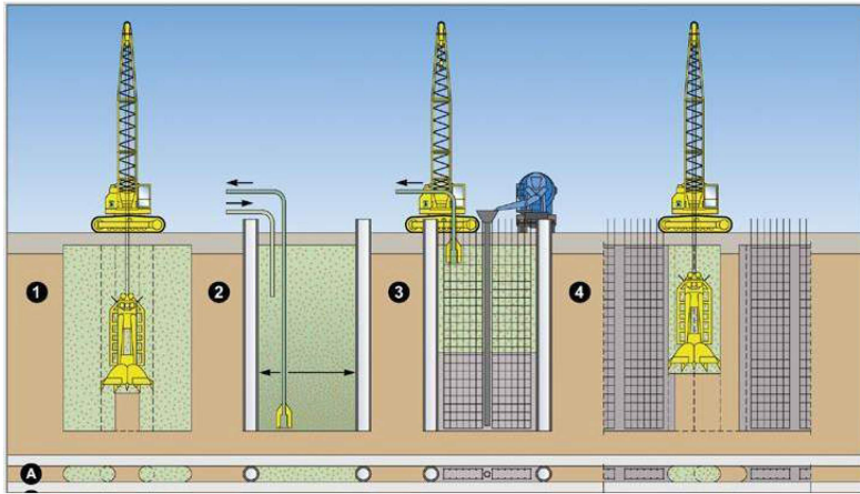
Schema Bauablauf Schlitzwandaufstellung
